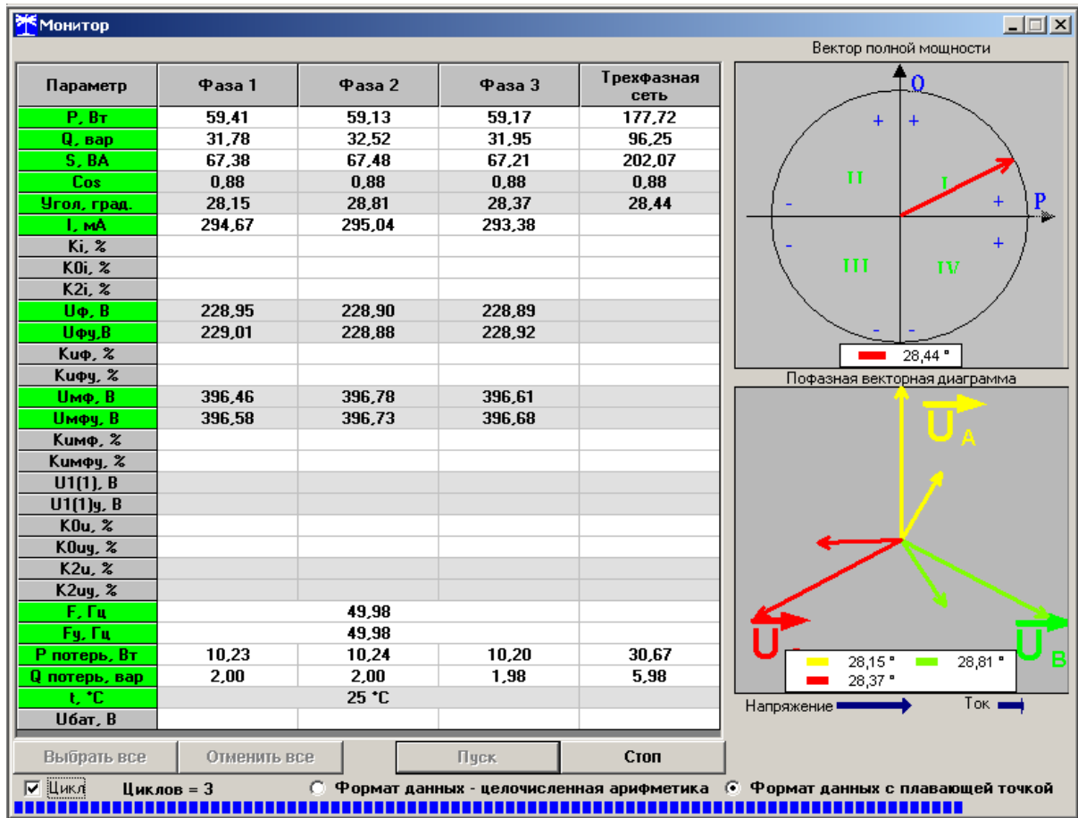
Рисунок 21 – Форма «Монитор»
