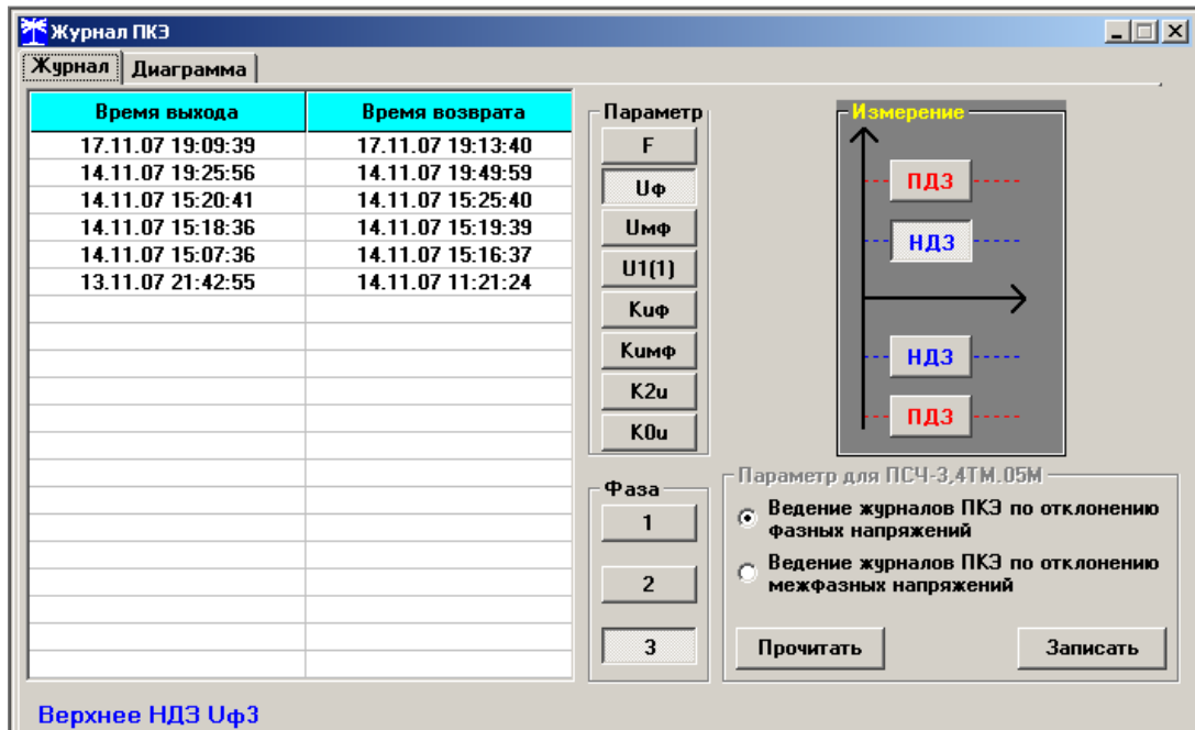
Рисунок 23 –Форма «Журналы ПКЭ» табличное представление
