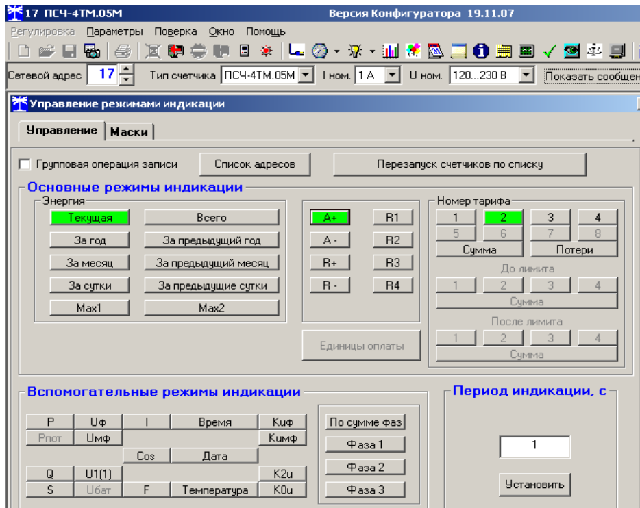
Рисунок 6 – Форма «Управление режимами индикации»
