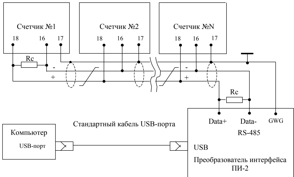
Схема подключения счетчиков к компьютеру
