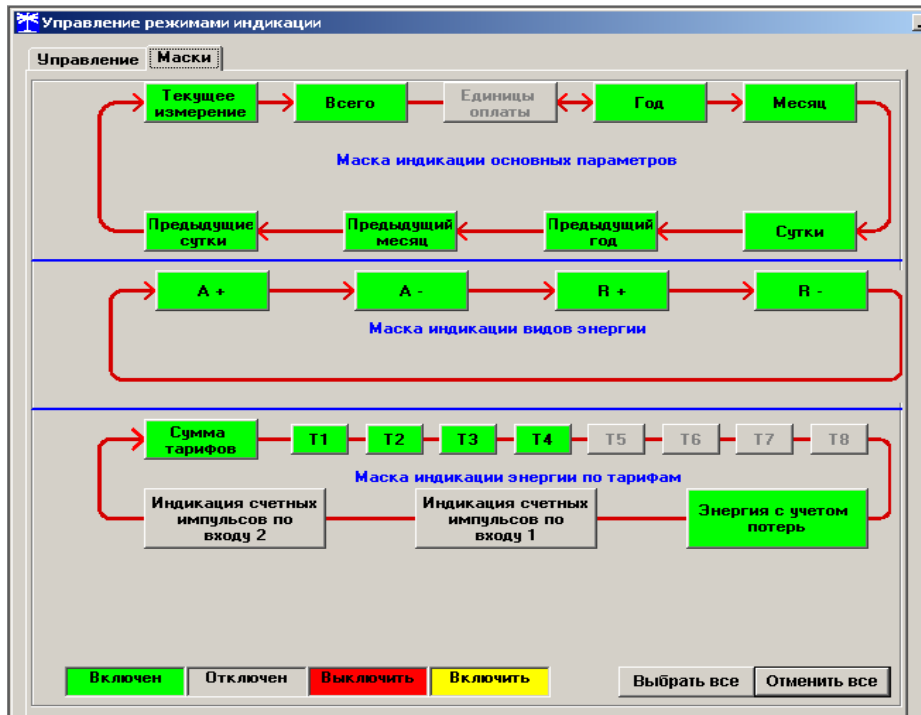
Рисунок 7– Вкладка «Маски» режимов индикации
